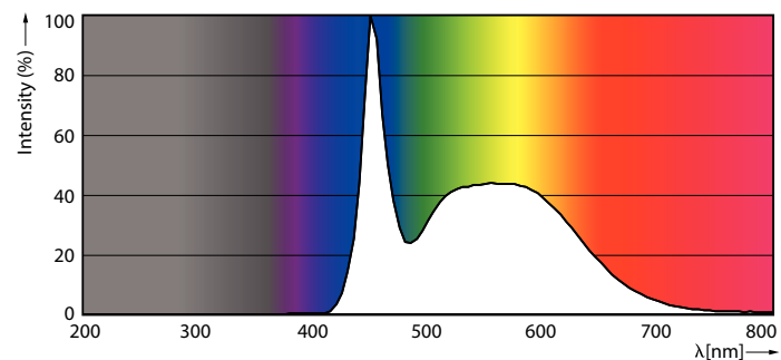
LEDtube_18W_G13_2100lm_865
